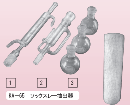
KA-65 4 円筒ろ紙
